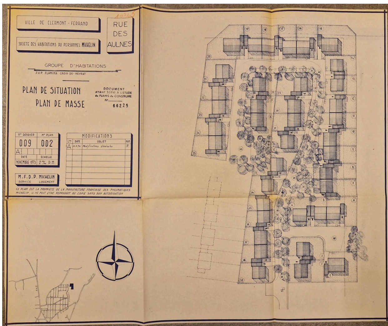
Projet de lotissement en mode Castor, rue des Aulnes : plan de situation et plan masse, 1973.
