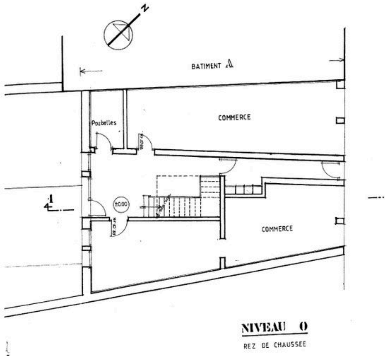
Plan du rez-de-chaussée / B. Verrier, I. Gaillard, 7 juin 1990. Ech. 1 : 100
