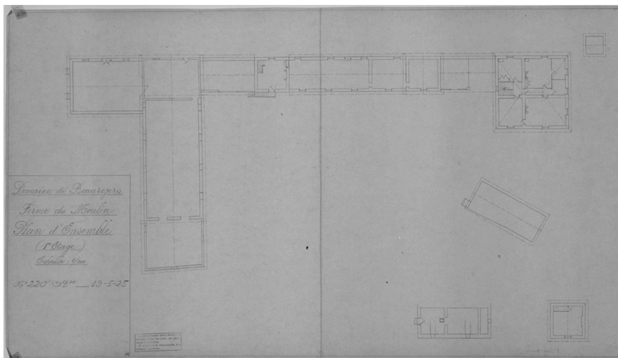
Domaine de Beaurevers. Ferme du Moulin. Plan d'ensemble (1er étage). 19 mai 1925.
