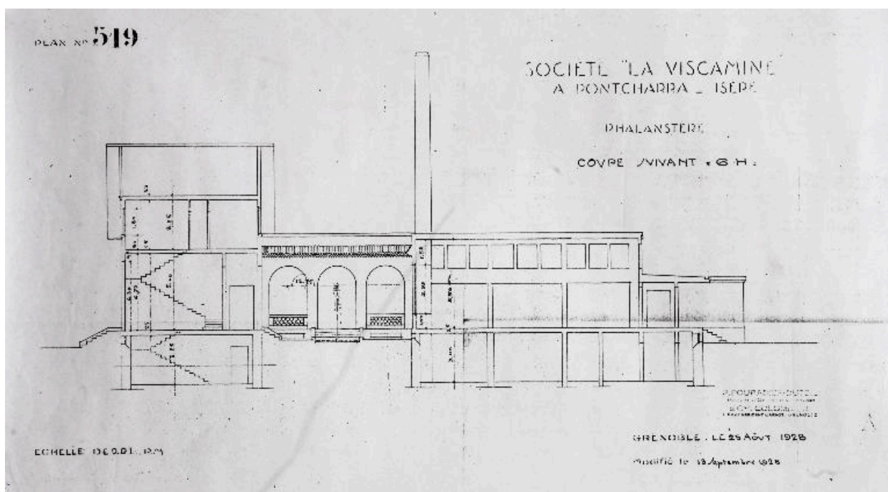
Phalanstère. Coupe suivant GH (1928)
