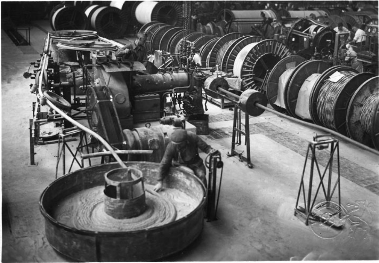
Chaîne de vulcanisation sur plateau, atelier qui n'existe plus aujourd'hui, archive privée de la société Nexans
