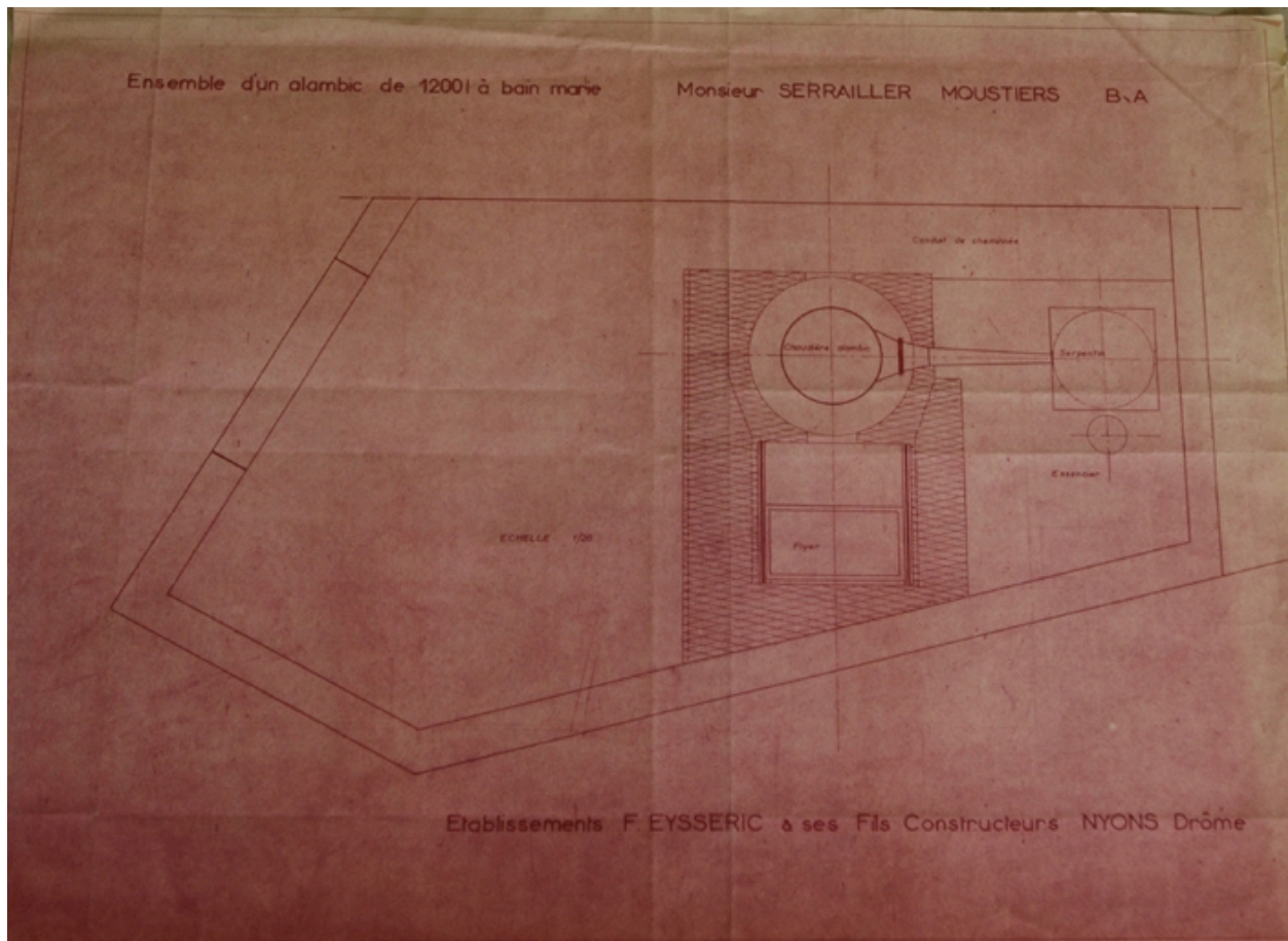
Ensemble d'un alambic de 1200litres (archives privées)
