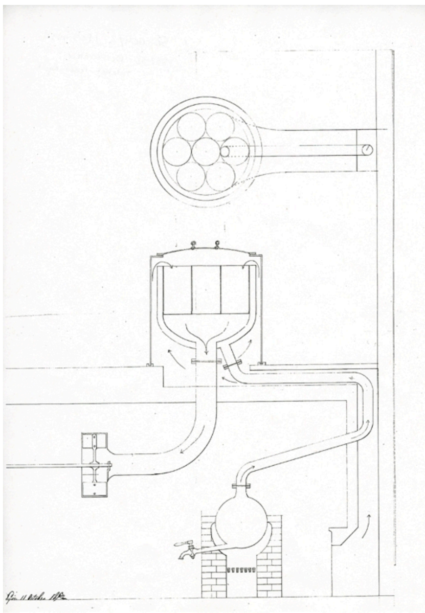
Schéma du dessiccateur Talabot-Persoz-Rogeat, 1856
