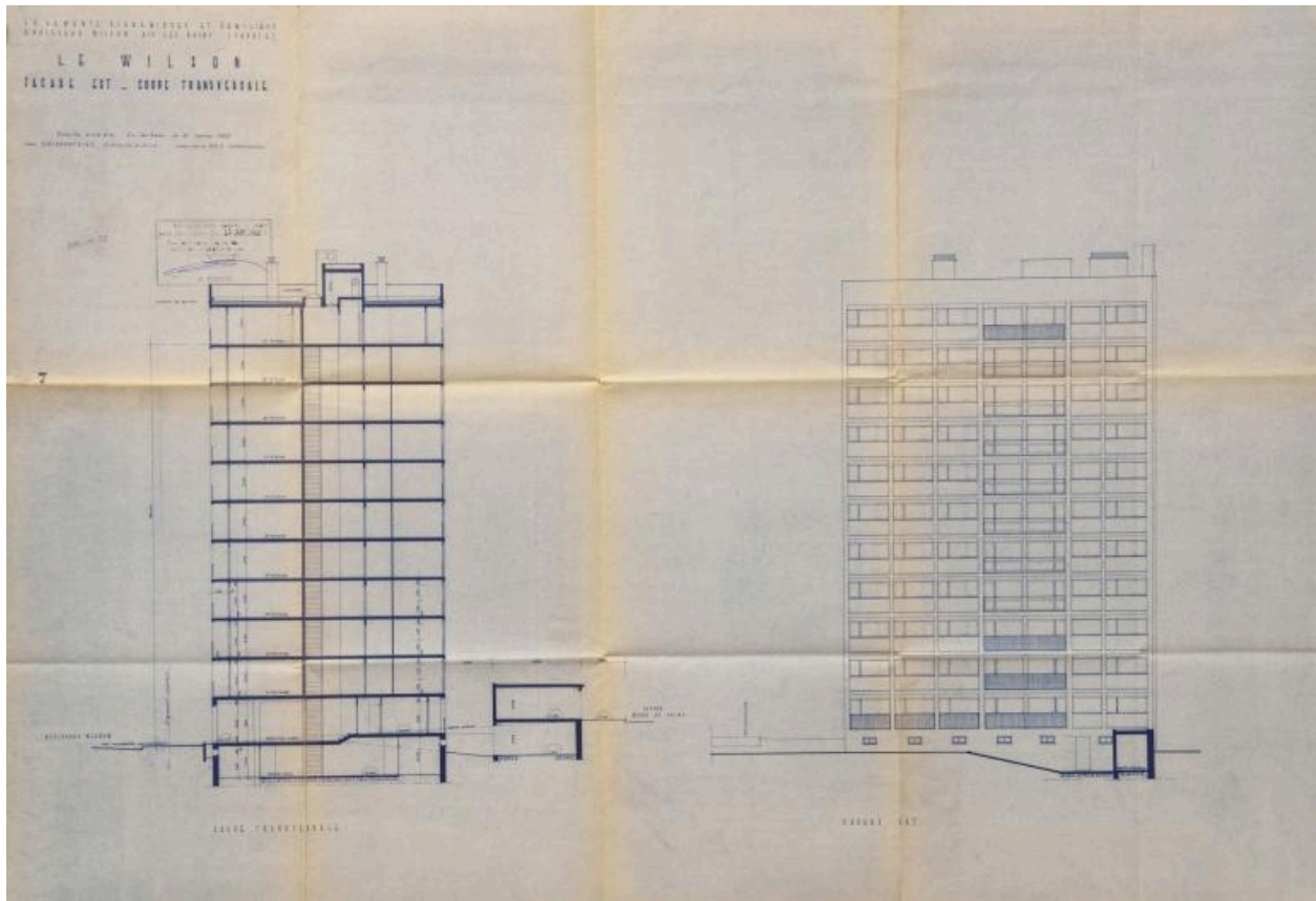
Coupe transversale et façade est, 1962
