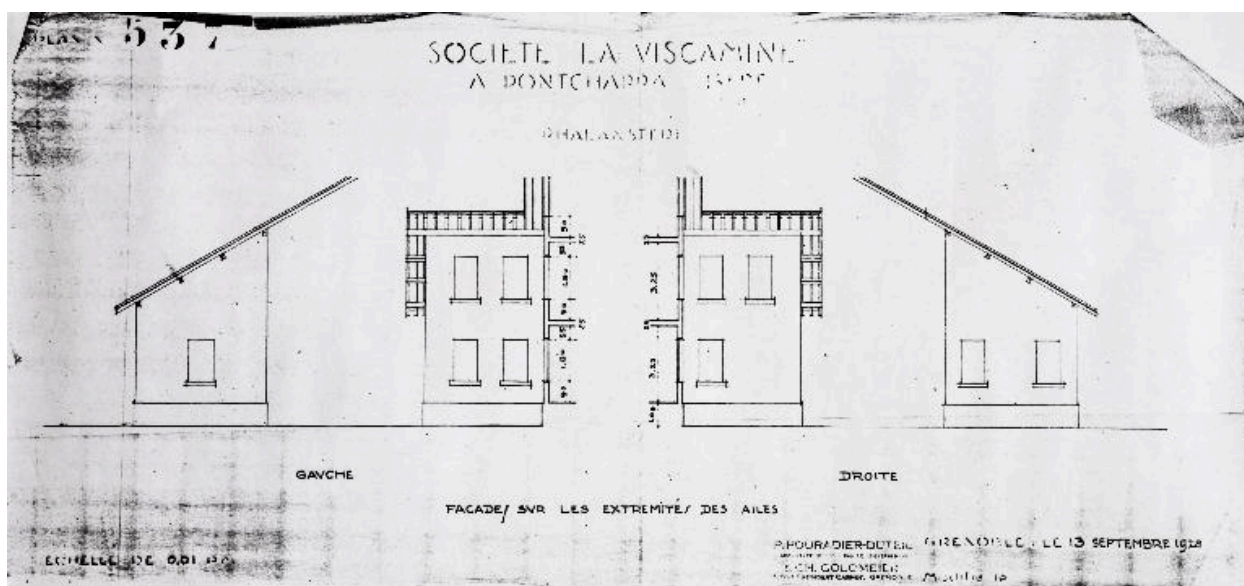
Phalanstère. Façades sur l'extrémité des ailes (1928)
