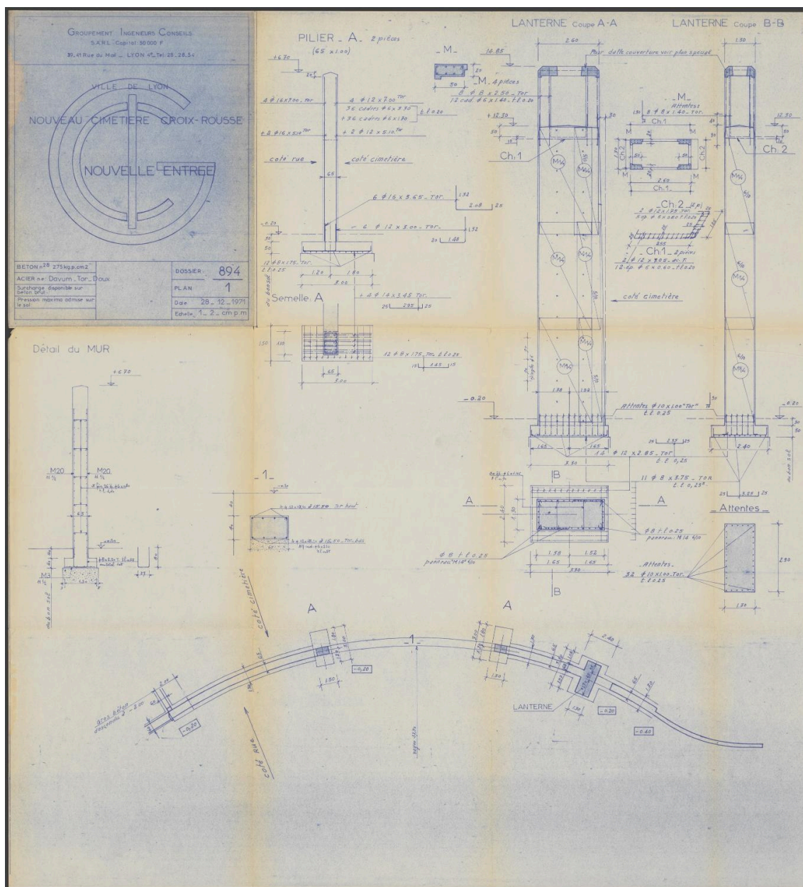
Plans et coupes cotés du mur, des piliers et de la lanterne, Groupement Ingénieurs Conseils, 1971
