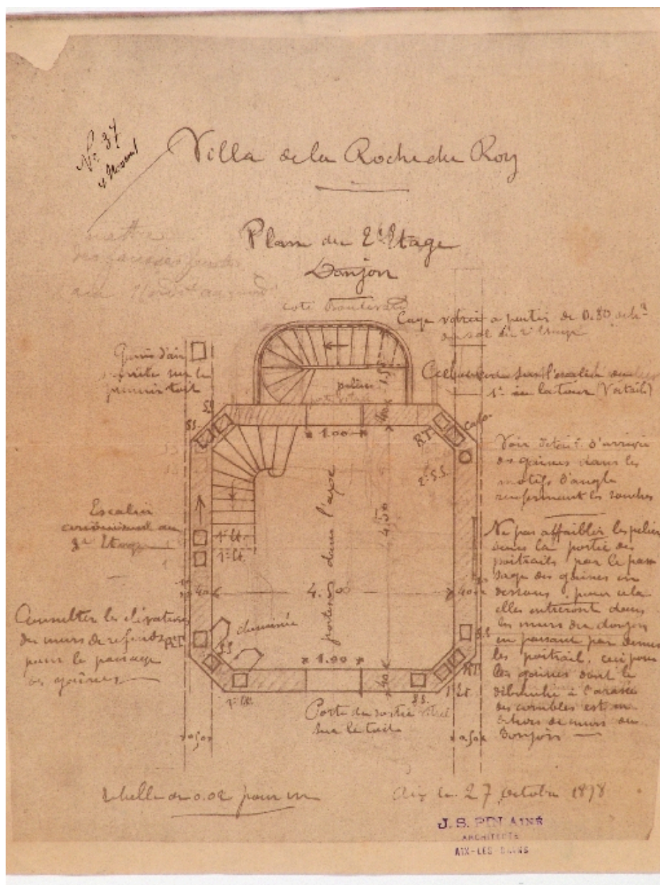
Plan du 2e étage du donjon
