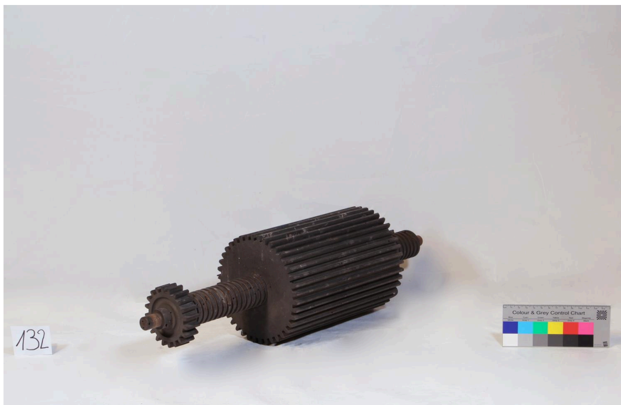
Engrenage (liste supplémentaire n°132), vue de côté
