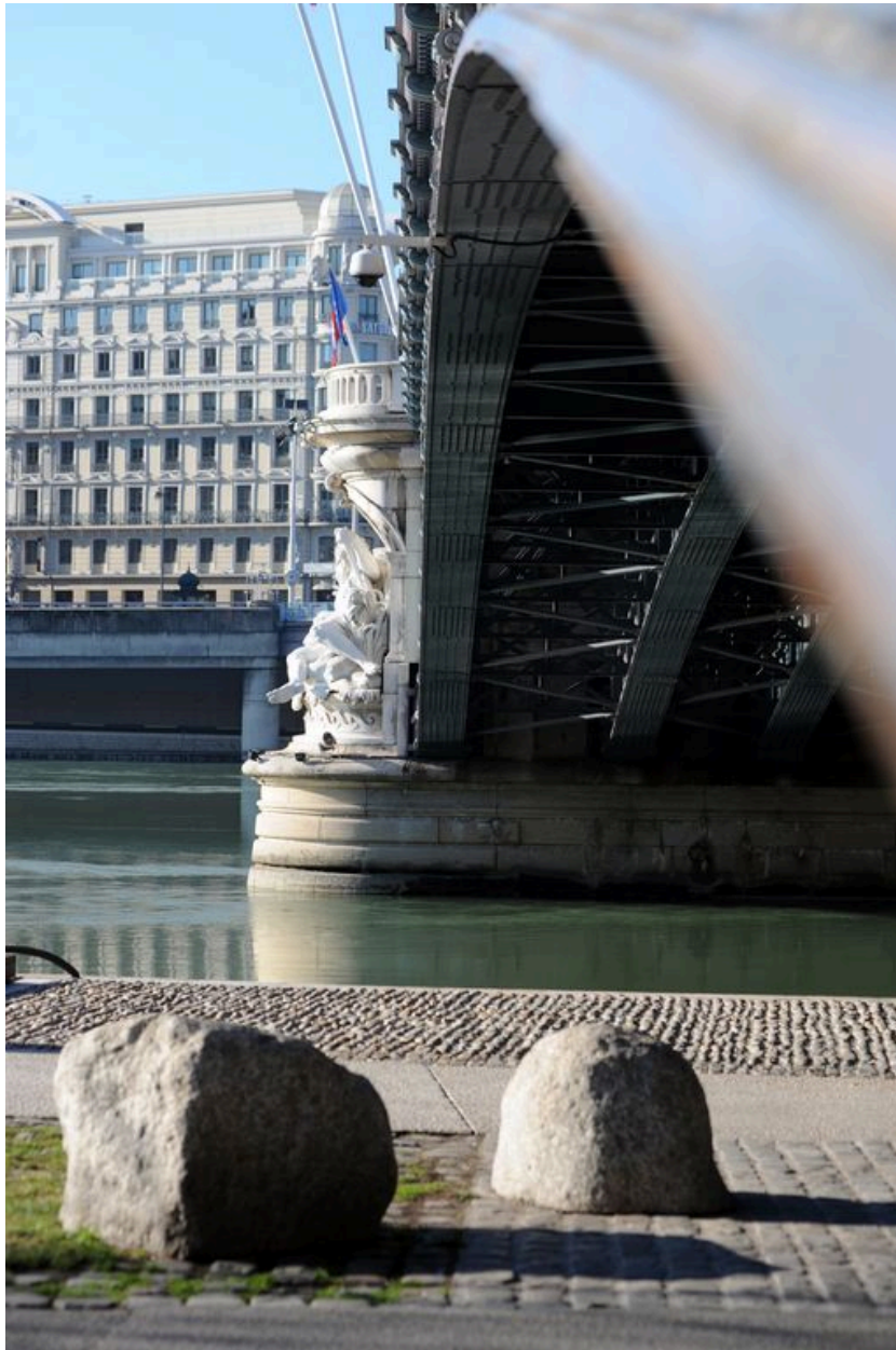
Arche gauche, face aval, de dessous, vue partielle : moitié gauche (depuis la rive droite)
