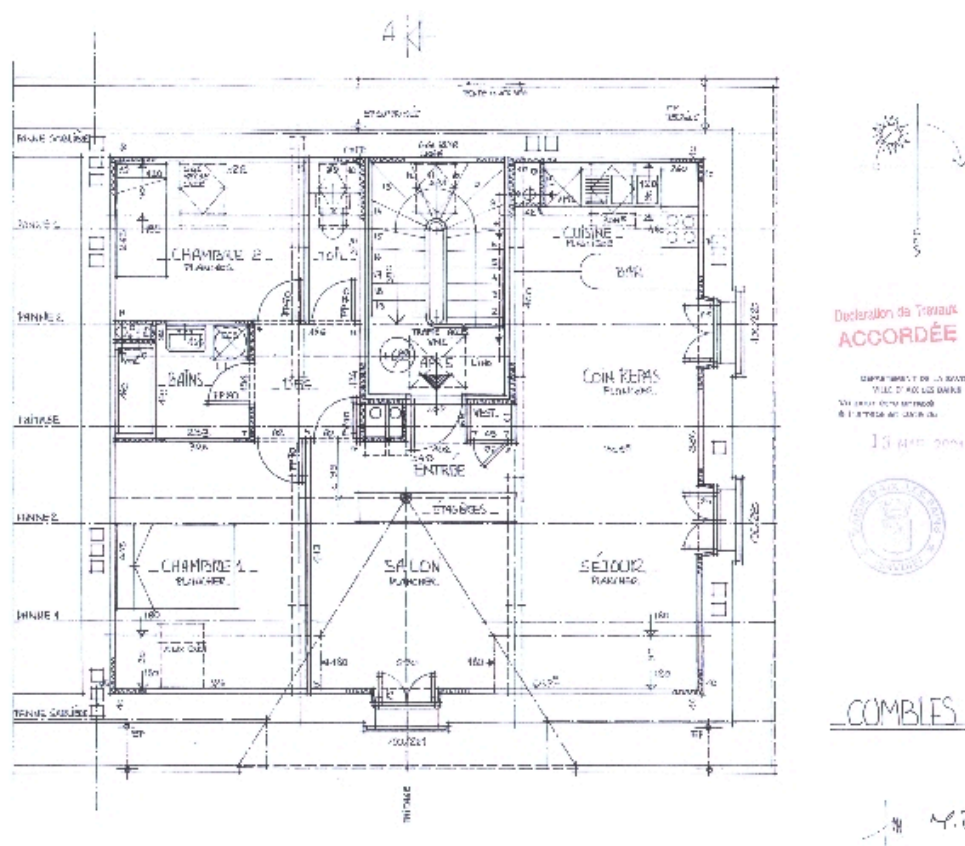
Plan des combles, 2000
