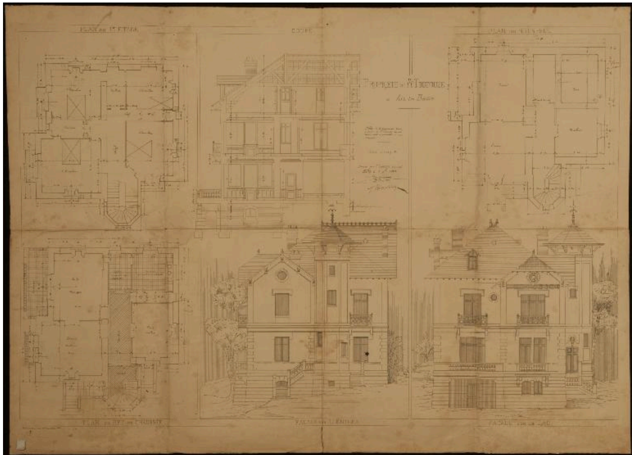
Plans, façades et coupe
