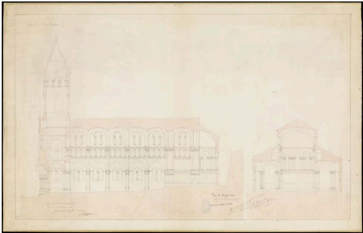
Coupes dressées par G. André pour C. Tisseur, 1874 (Arch. mun. Lyon, 2 S 00231/3, dessin (encre et lavis).
