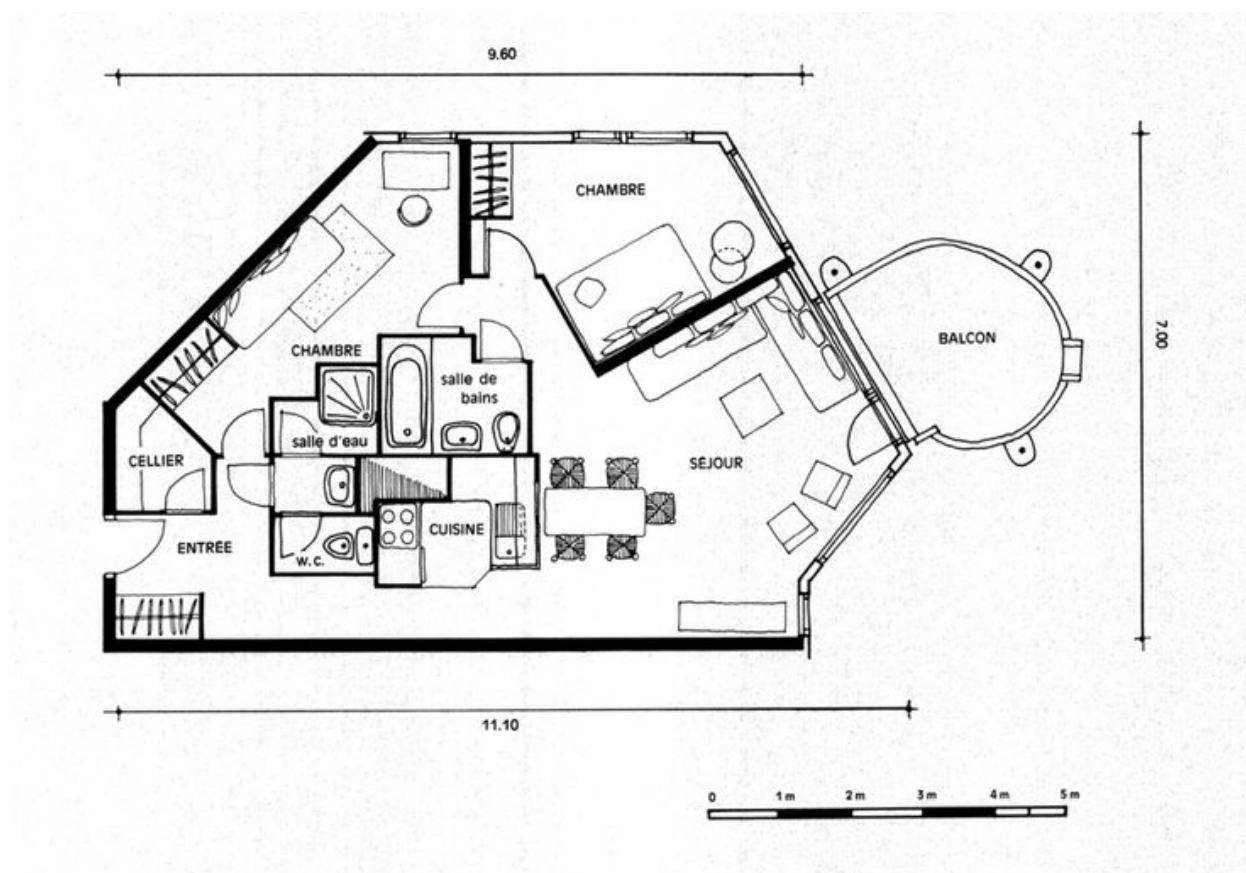
Plan d'un appartement du 6e niveau
