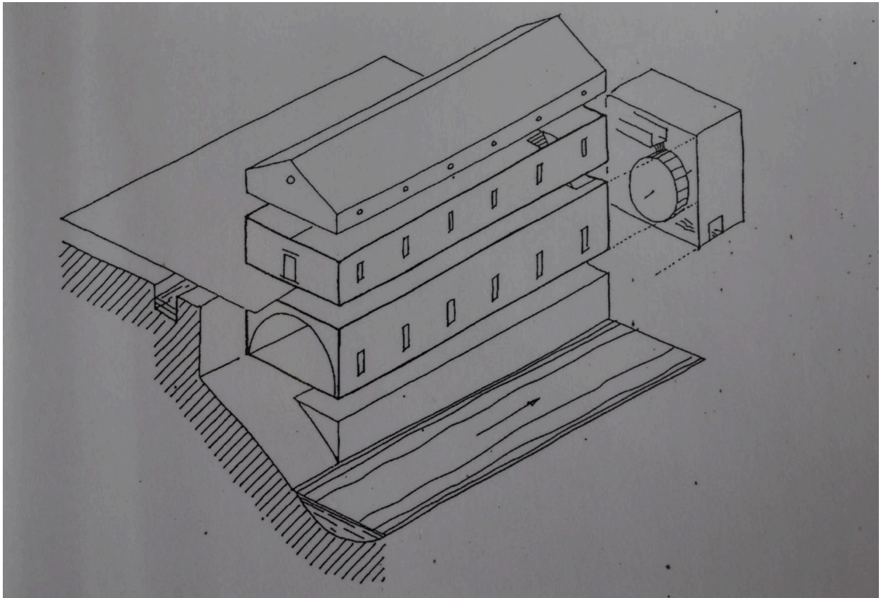
Coupe axonométrique du moulinage (ENSAL)
