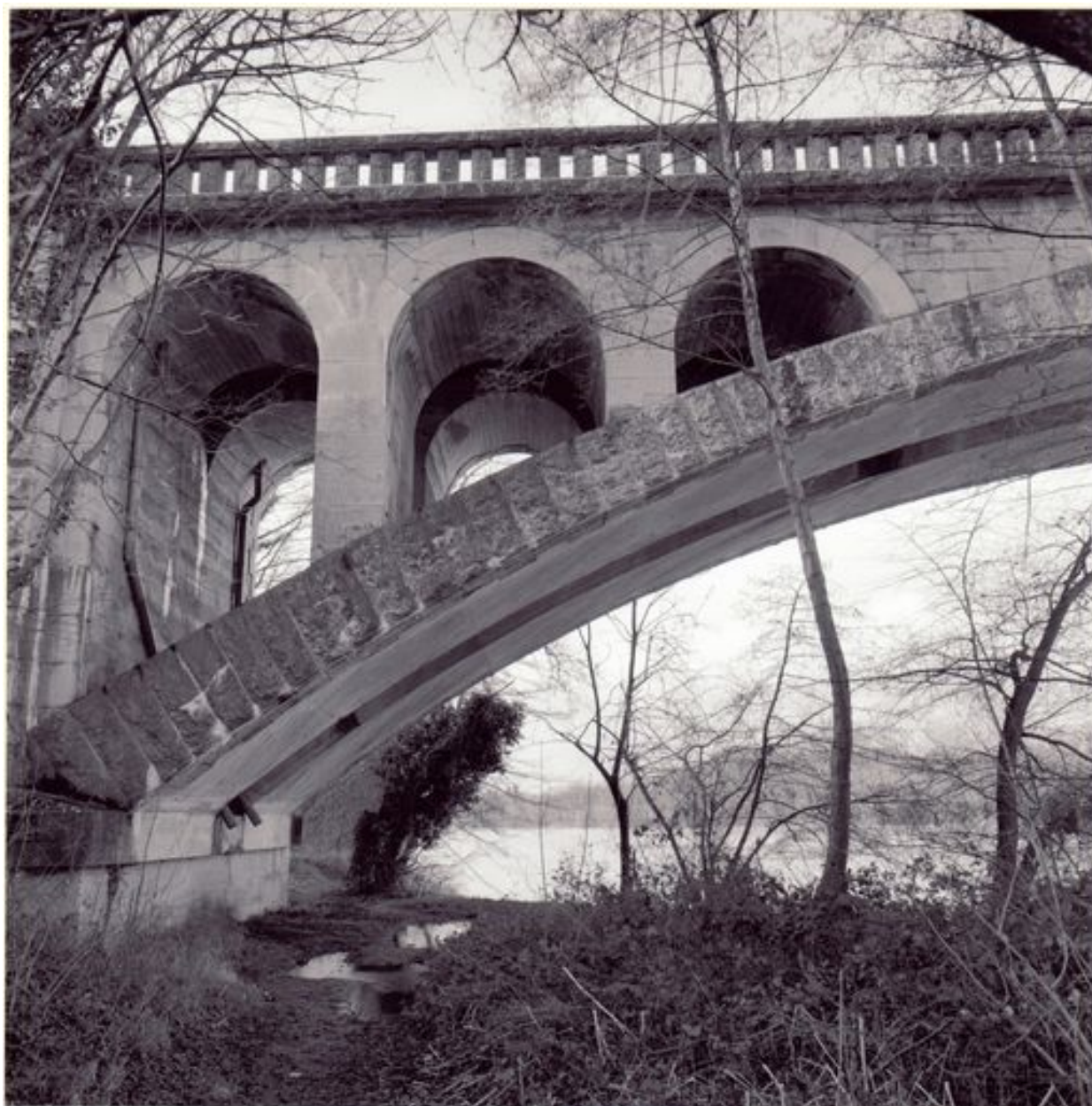
Détail du départ de la 1ère arche, côté sud
