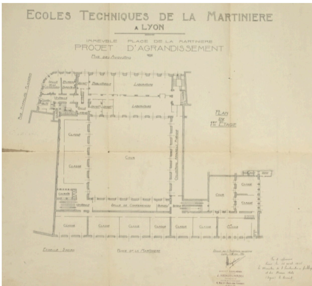
Ecoles techniques de la Martinière, projet d'agrandissement, plan du 1er étage, 31 mai 1924. Document figuré. Plan, élévation. 31 mai 1924. 1:100. Fondation Martin. non coté
