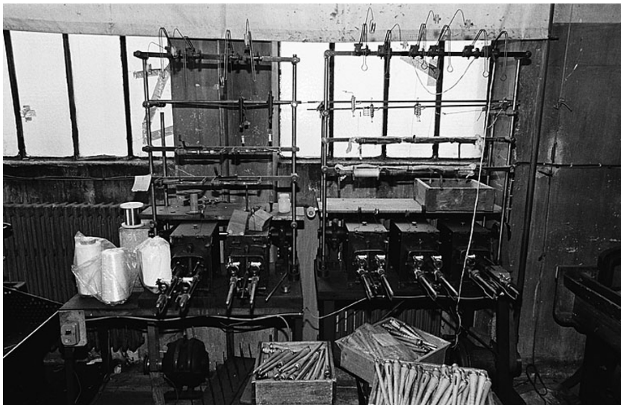
Deux petites cannetières dites productive C, à 4 et 6 broches montées sur un plateau en bois dur
