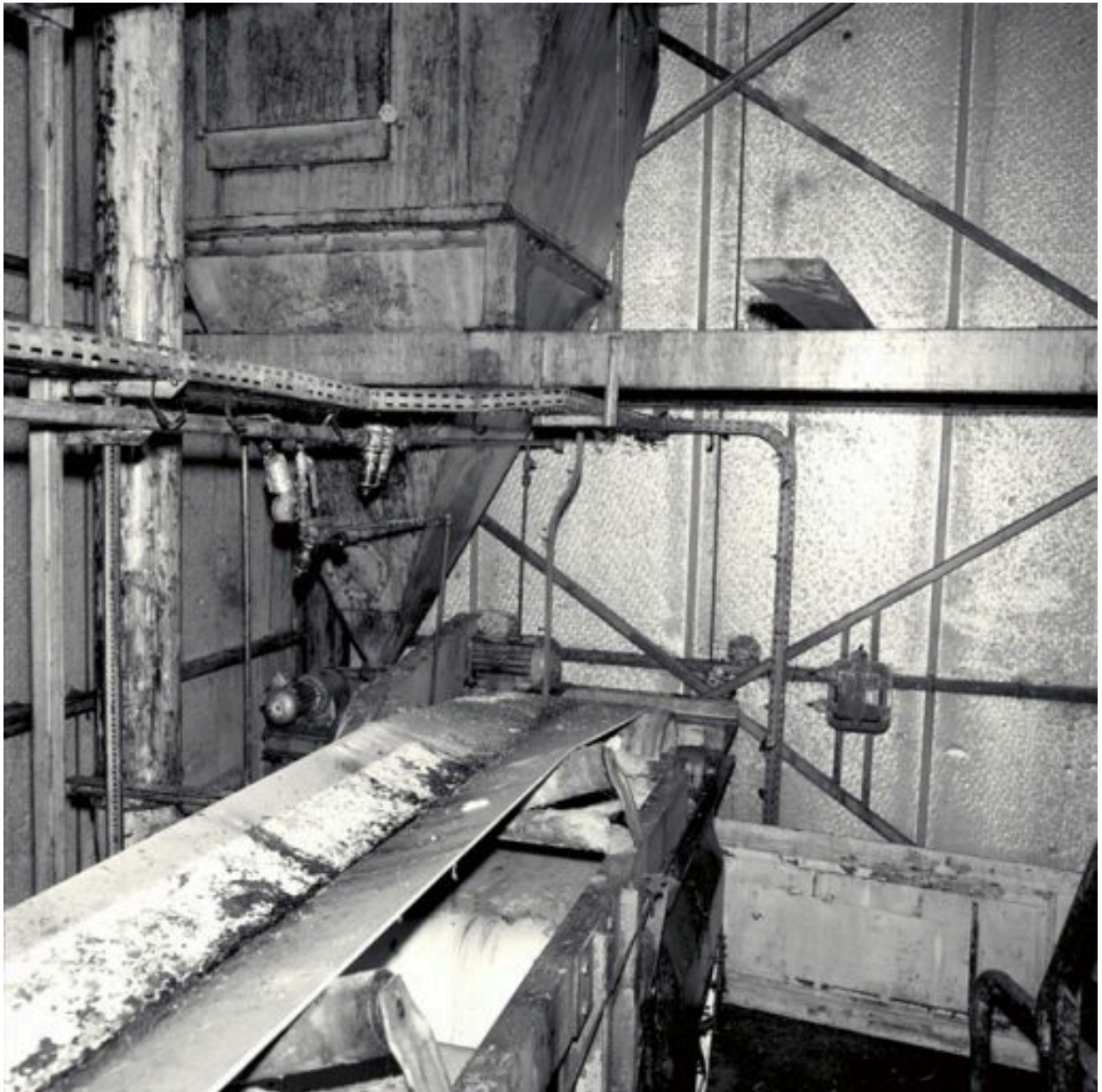
La trémie à l'extrémité du transporteur à bande
