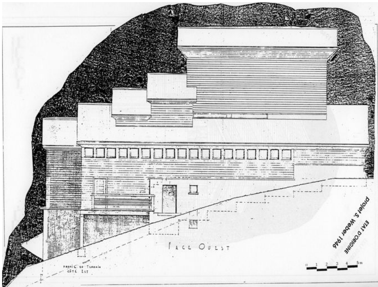
Gare supérieure. Elévation ouest. Projet / Stéphane Weber, 1946
