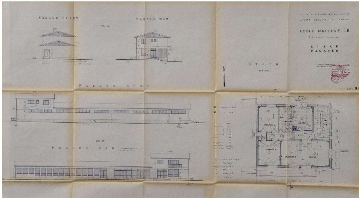
Plan et élévations, 1966
