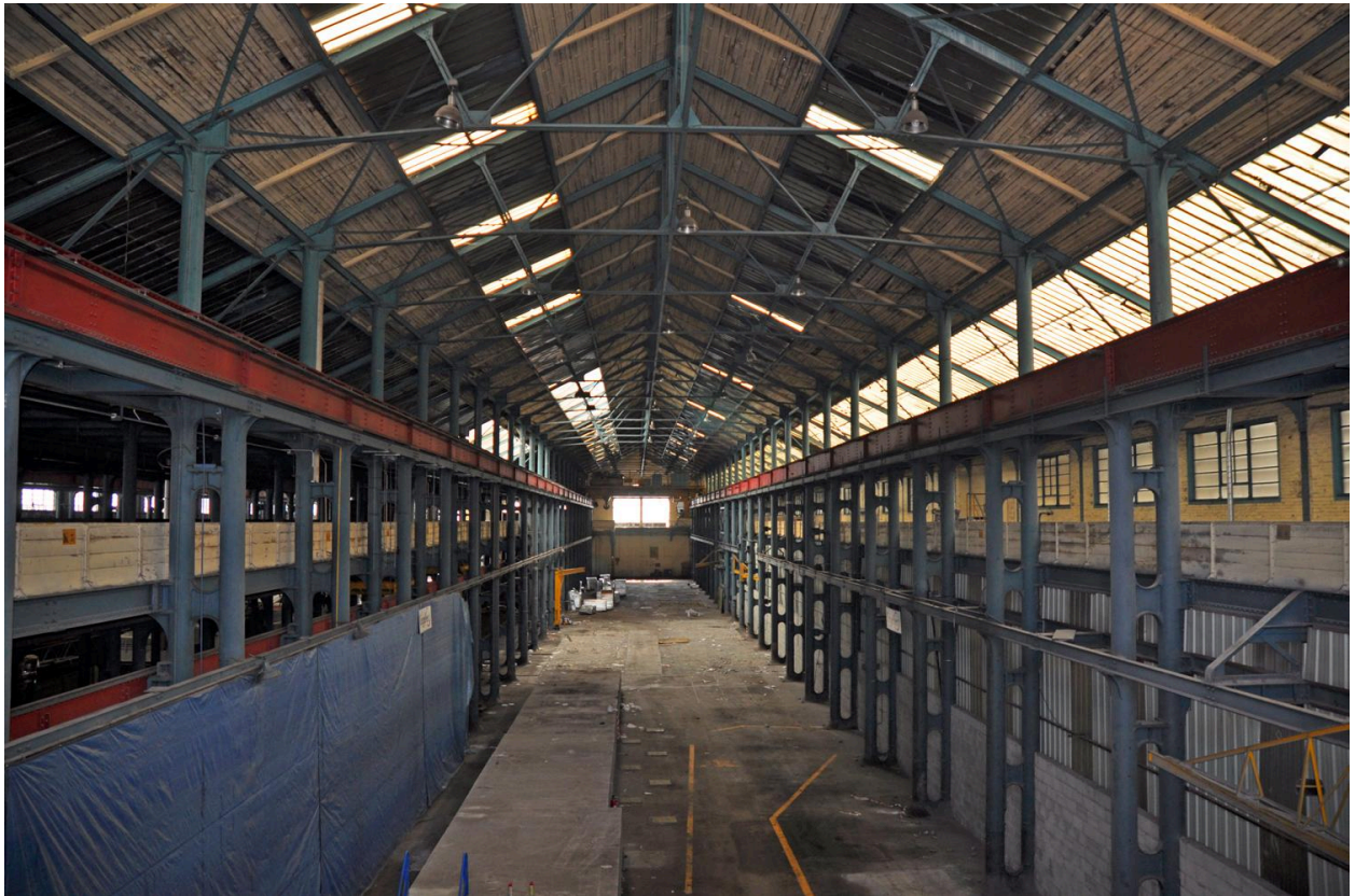
Vue d'ensemble de la charpente métallique de la Halle 07
