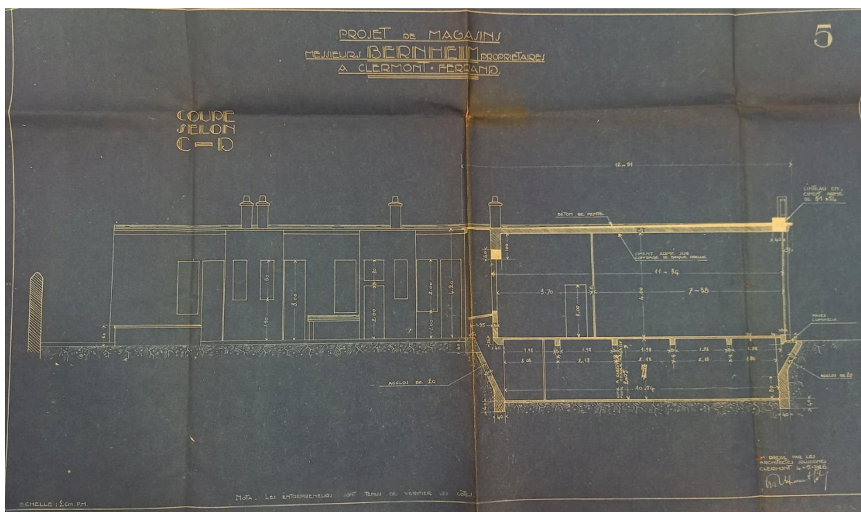
Coupe nord-sud, 21 avenue Charras
