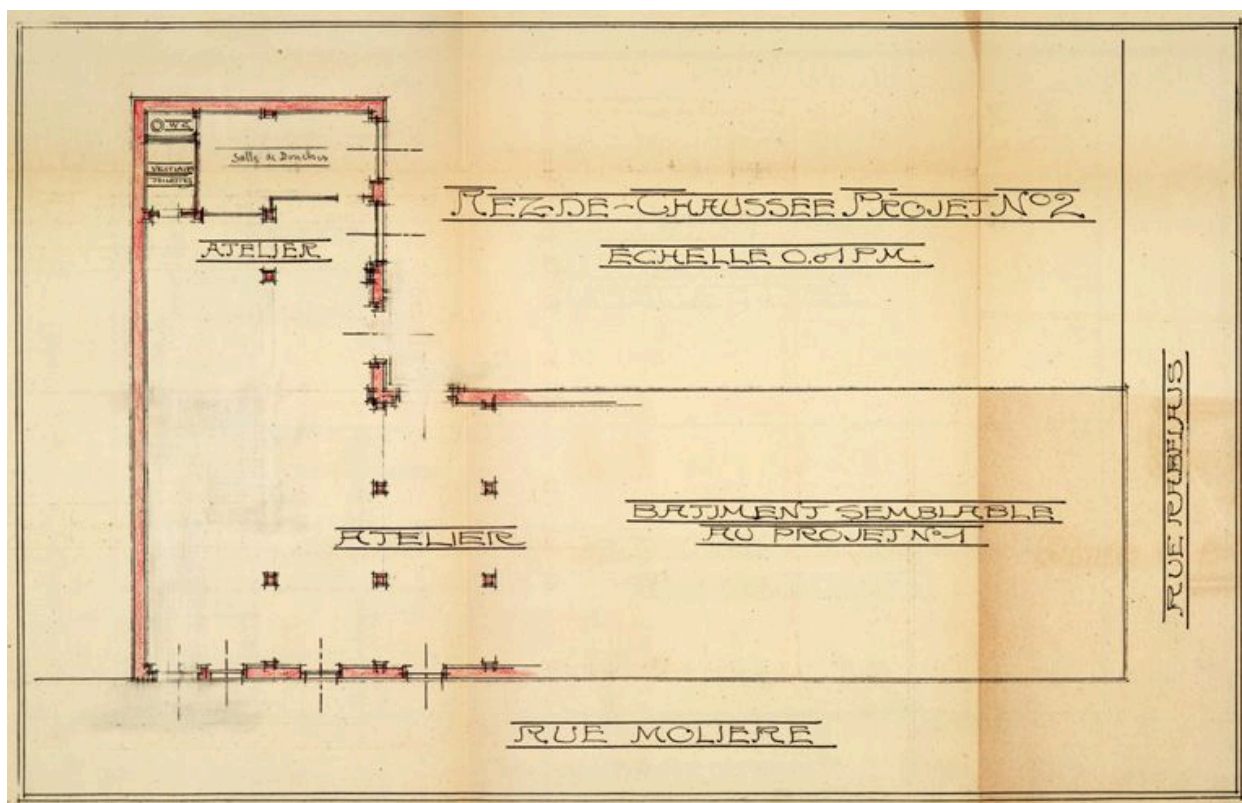
Rez-de-chaussée projet n°2
