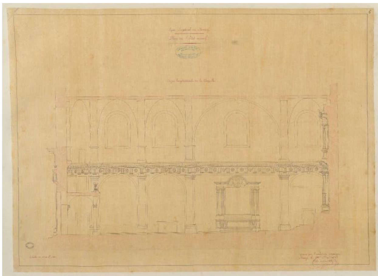
Coupe longitudinale en 1861, par Ch. Martin (AN F/17/*/2435)
