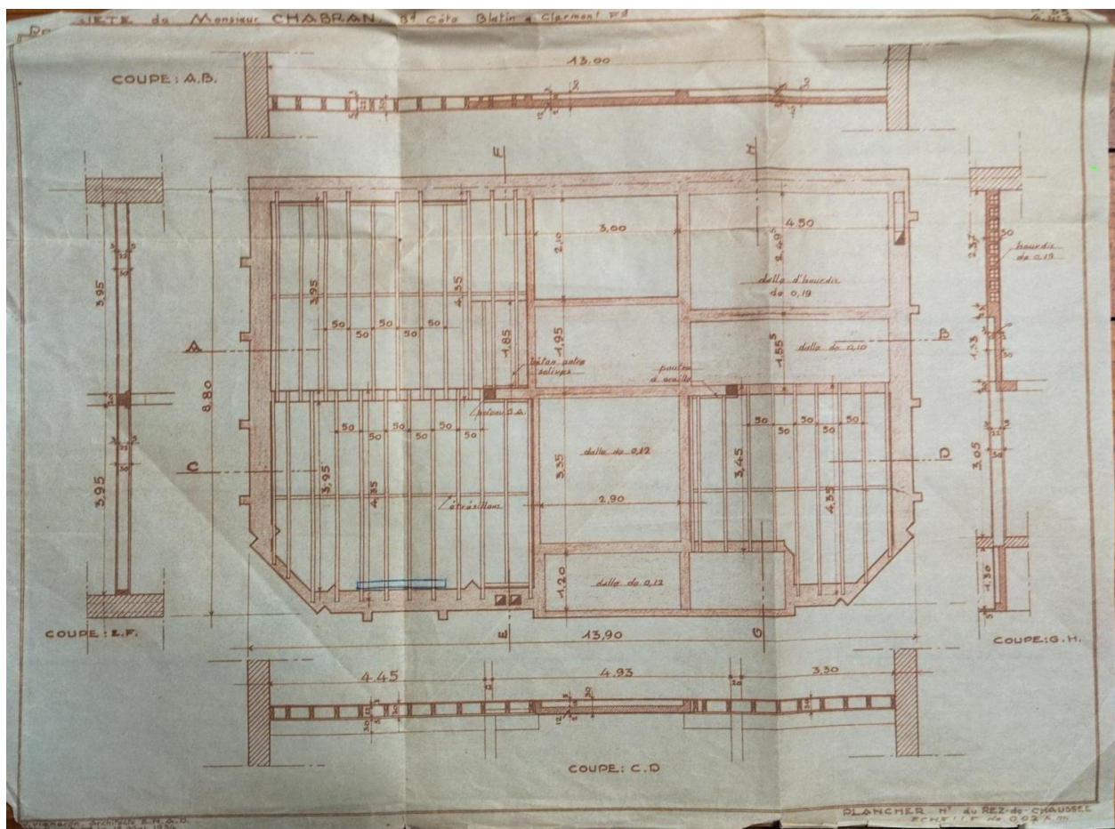
Plan de couverture (plans modificatifs 1934)
