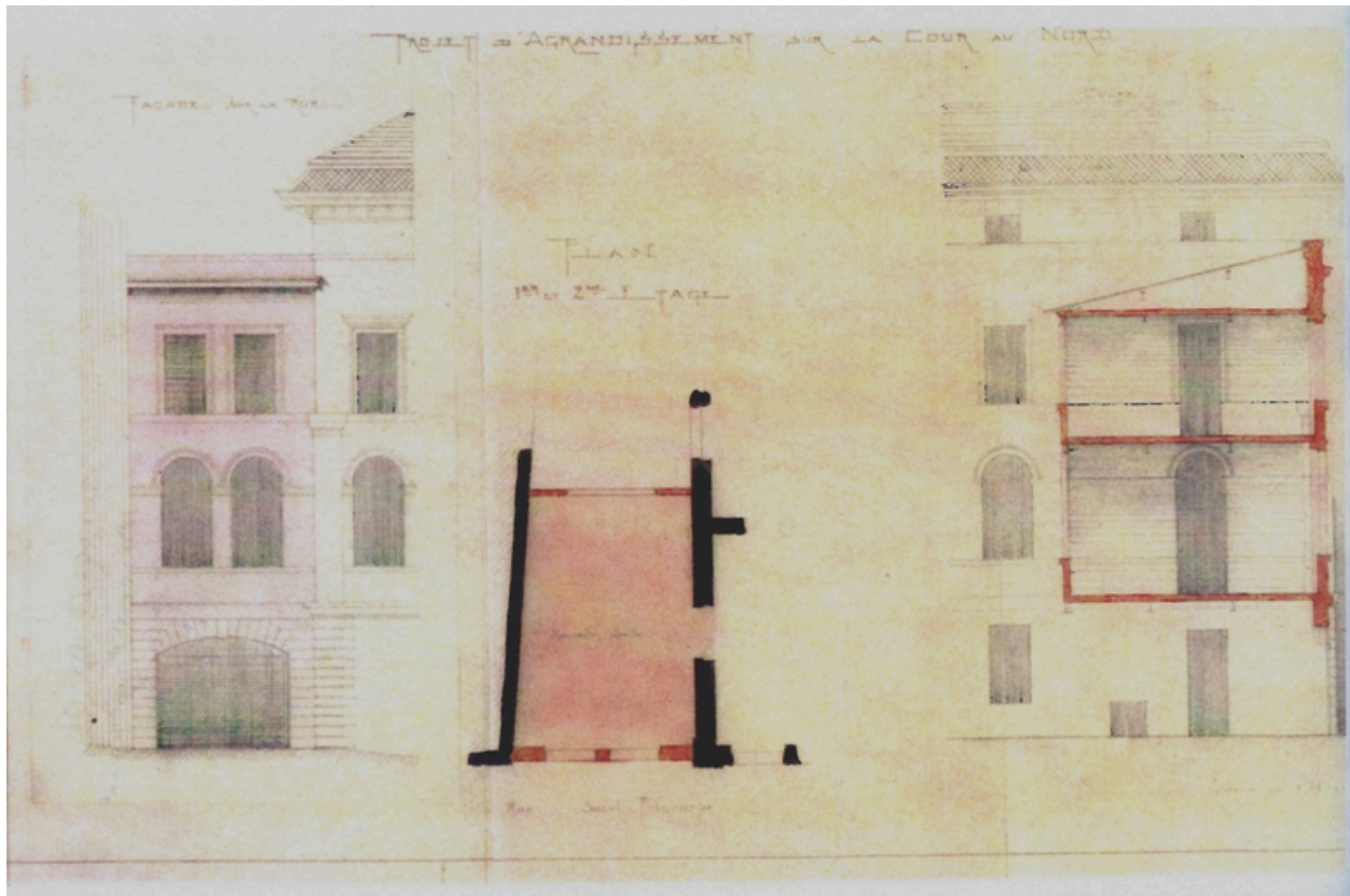
Projet d'agrandissement sur la cour au nord, façade sur rue, plan 1er et 2ème étages, coupe, 1898
