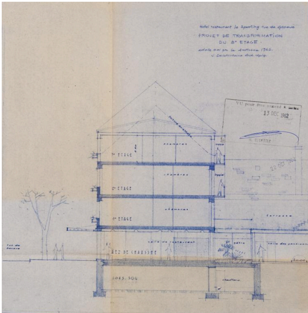
Hôtel le Sporting : projet de transformation du 3e étage, coupe, 1962
