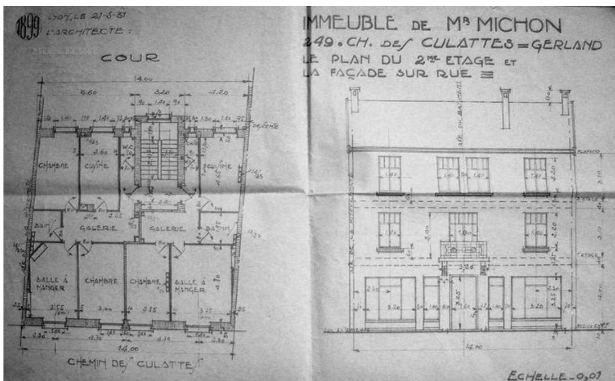
Plan du 2eme étage et façades, Immeuble de Monsieur Michon à Gerland à Gerland, 249 rue des Culattes, 21 mai 1931 par Pierre Renaud architecte, échelle 1/100. (Arch. mun. Lyon)
