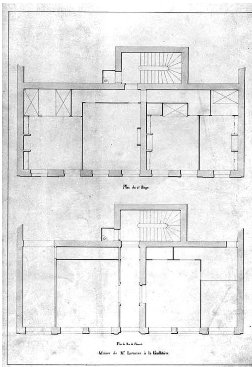
Plans de la maison de M. Laracine à la Guillotière / Feuga, 1919
