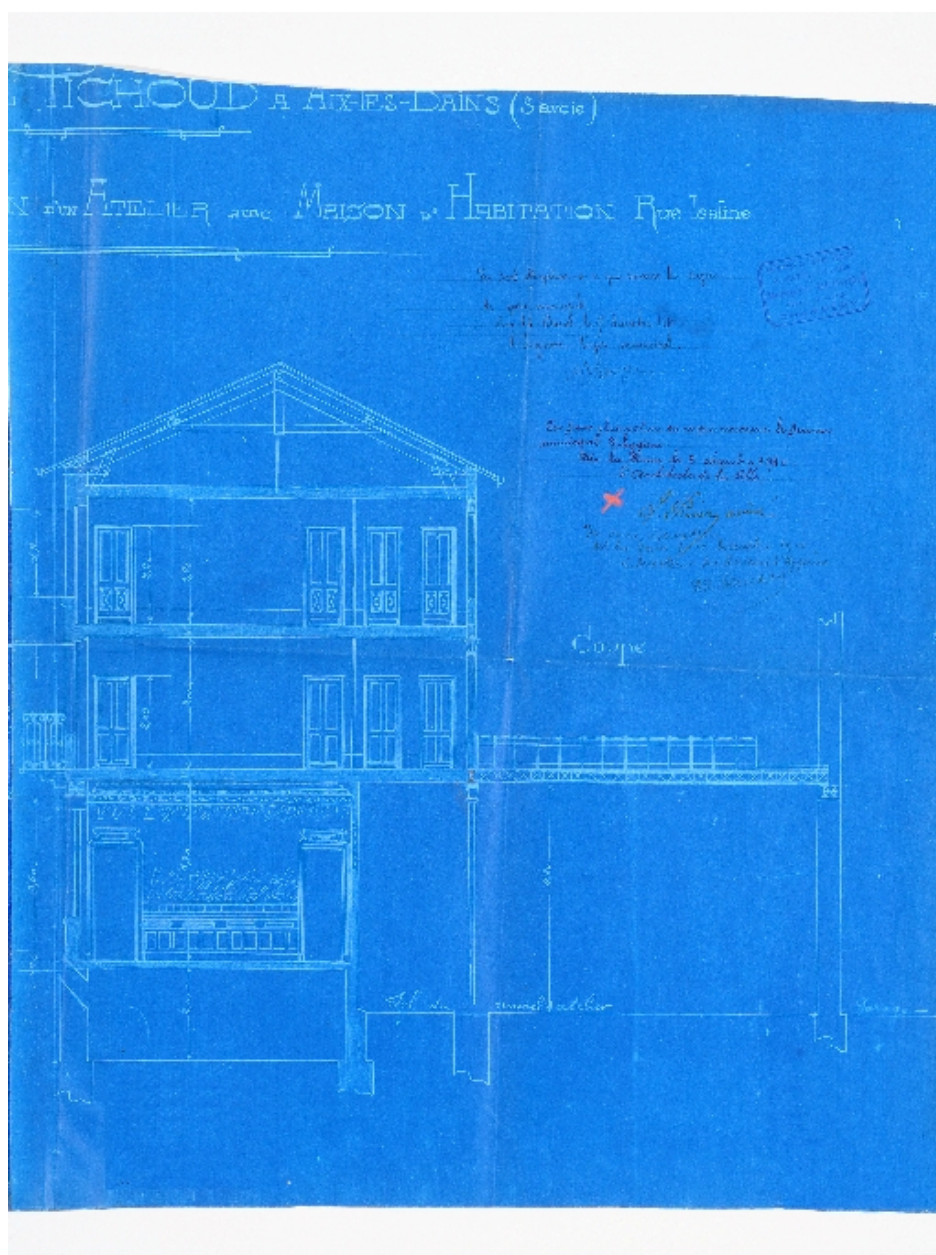
Coupe transversale
