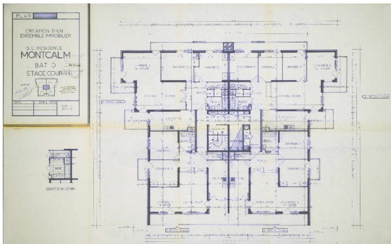
Bât. D : Plan d'un étage
