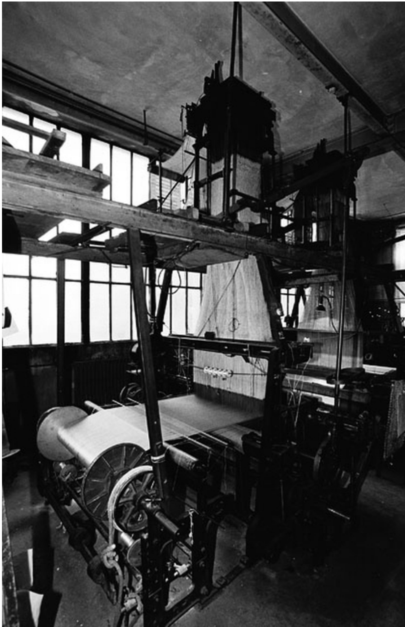
Métier à tisser jacquard, petit battant, à mécanique Verdol, de marque Diederich
