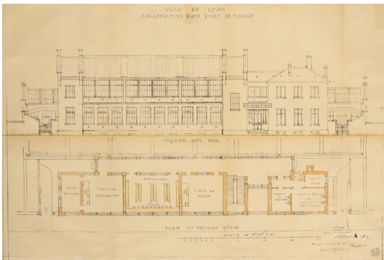
Ecole de tissage [Projet non réalisé]. 1905, plan du 1er étage et élévation de la façade. (AC Lyon. 2 S 00488 2)
