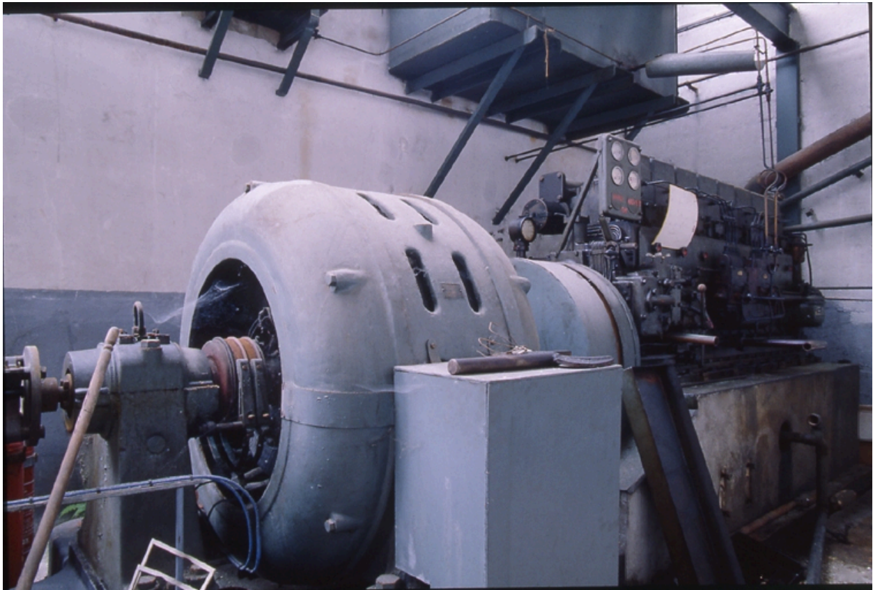
Chaudière-alternateur
