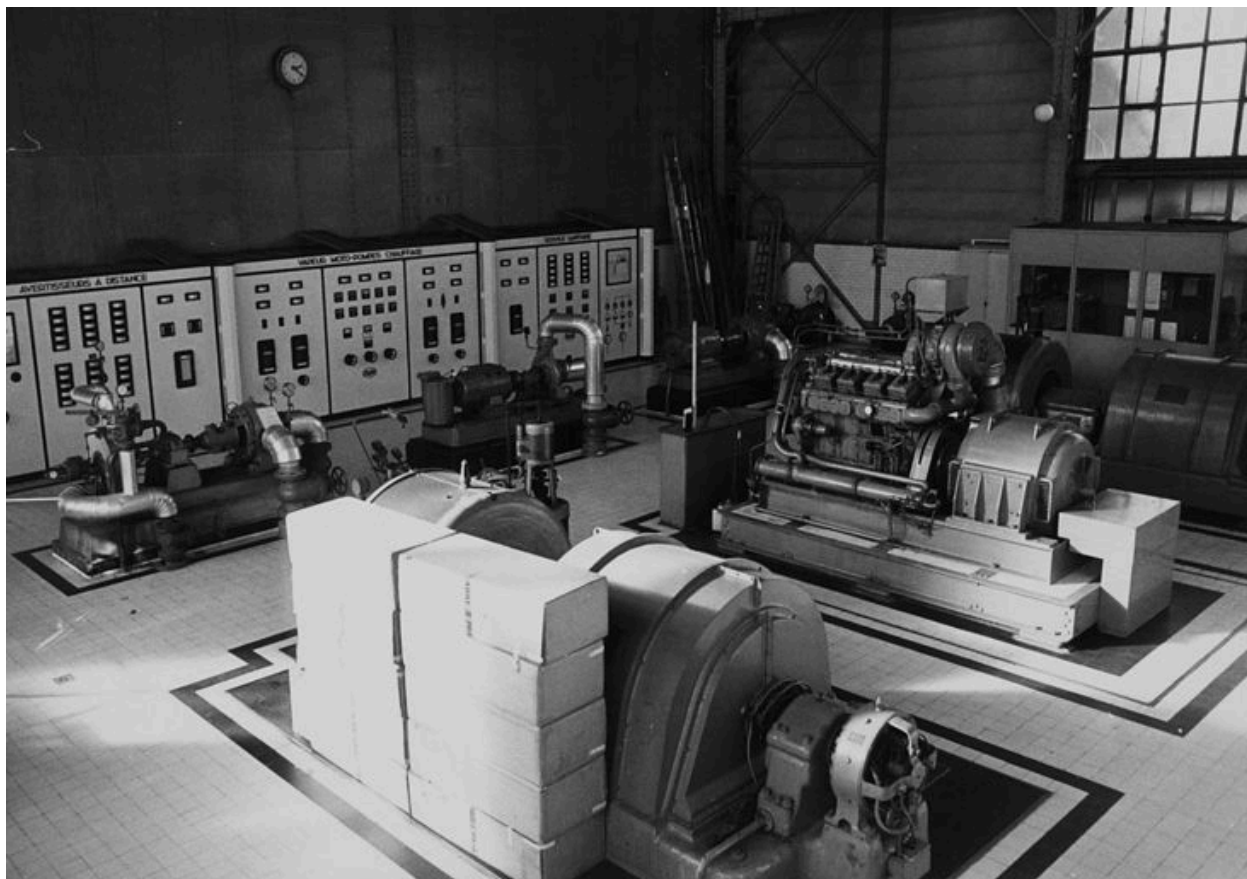
Centrale électrique. Tableau du service chauffage et du service sanitaire. Photogr., décembre 1972
