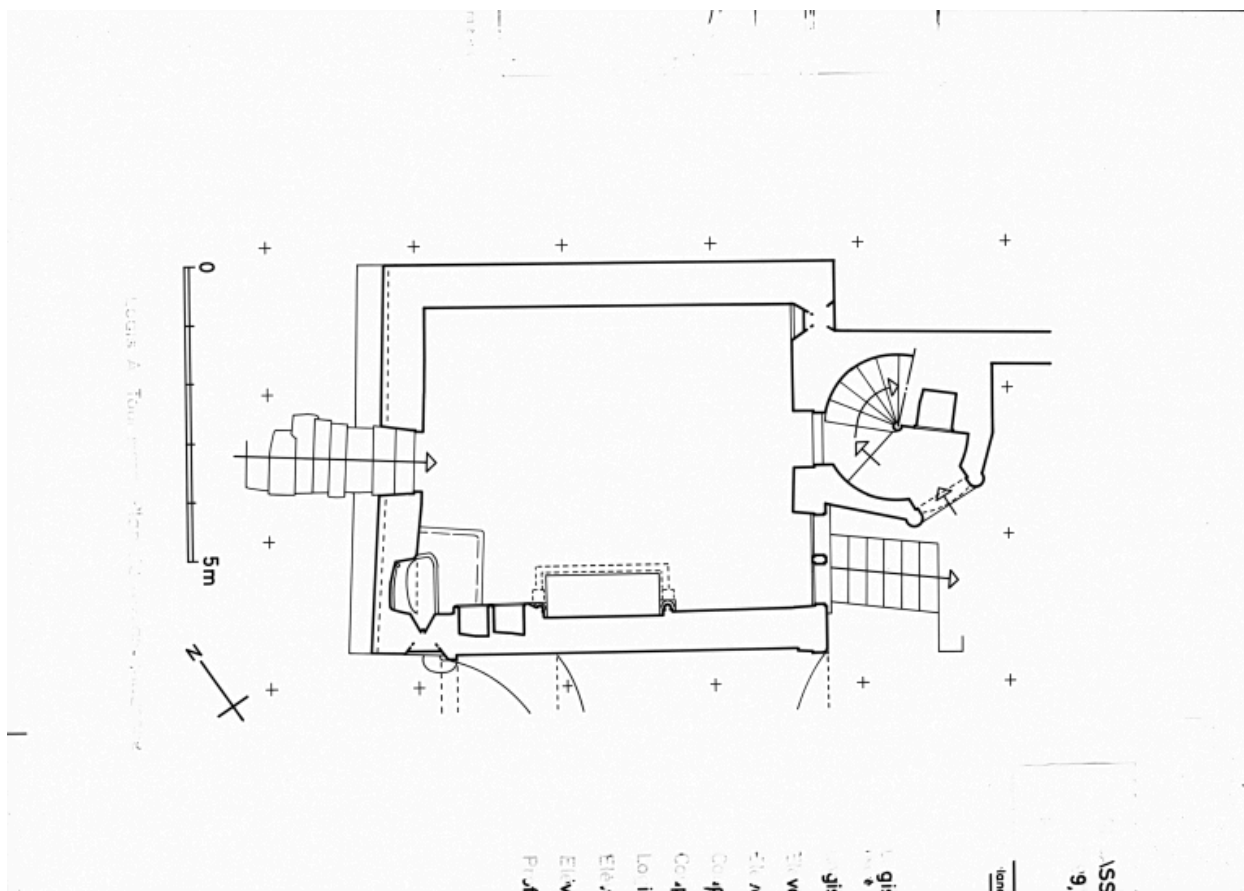
Tour nord, plan du rez-de-chaussée surélevé, Logis A, relevé expédié.
