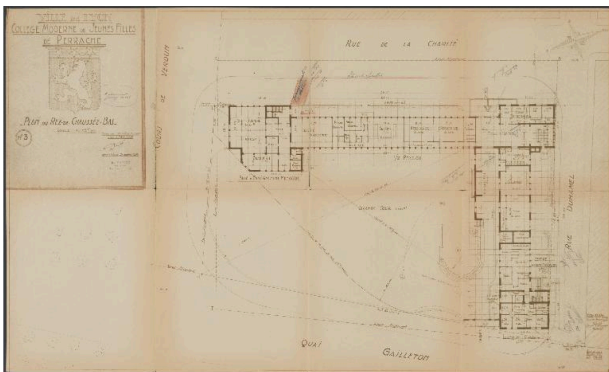
Plan du rez-de-chaussée bas, par E. Payen, 1954 (AC Lyon, 838 WP 001)
