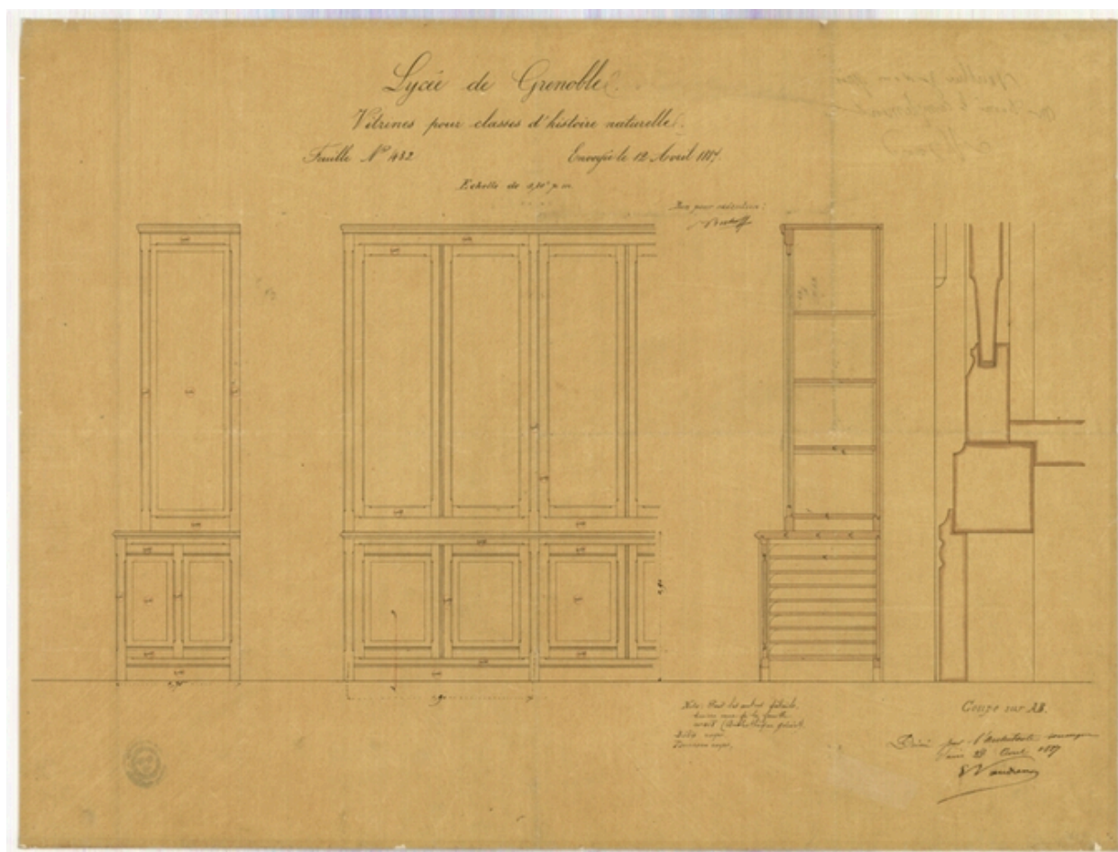
Plan. Vitrines pour les classes d'histoire naturelle. 12 avril 1887.
