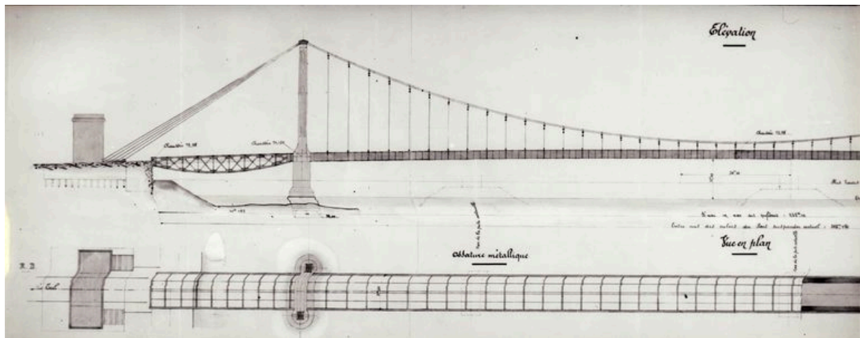
Ponts et chaussées... Reconstruction du pont du Teil sur le Rhône. Ensemble [partie gauche] / Compagnie Fives-Lille, 21 avril 1927 (AD Ardèche, 2S 30/11)
