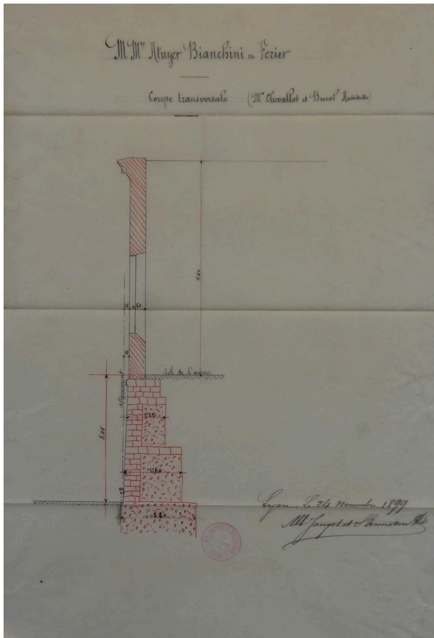
Coupe transversale usine 1899 (AC Lyon 314W138-218)
