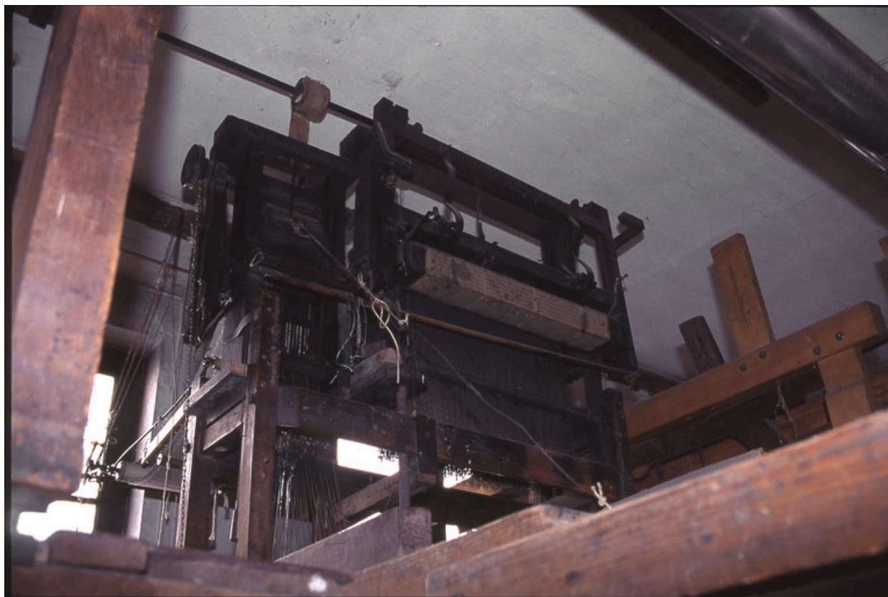
mécanique Jacquard de 1100 crochets
