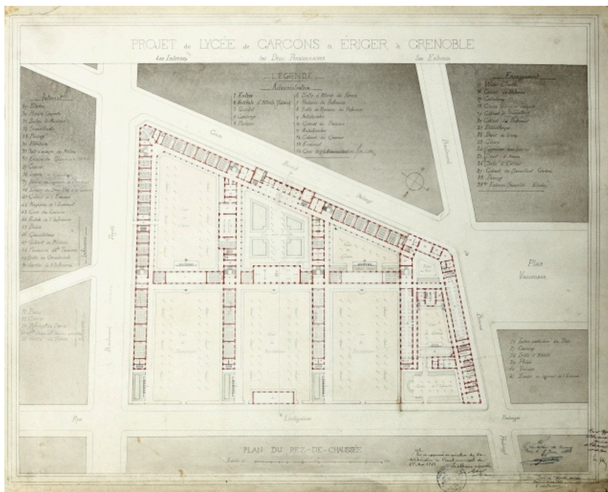
Projet de construction. Plan du rez-de-chaussée, 29 mars 1883. Document figuré. Plan. Aquarelle sur papier. 79 x 63 cm Archives municipales, Grenoble. 2 Fi 300
