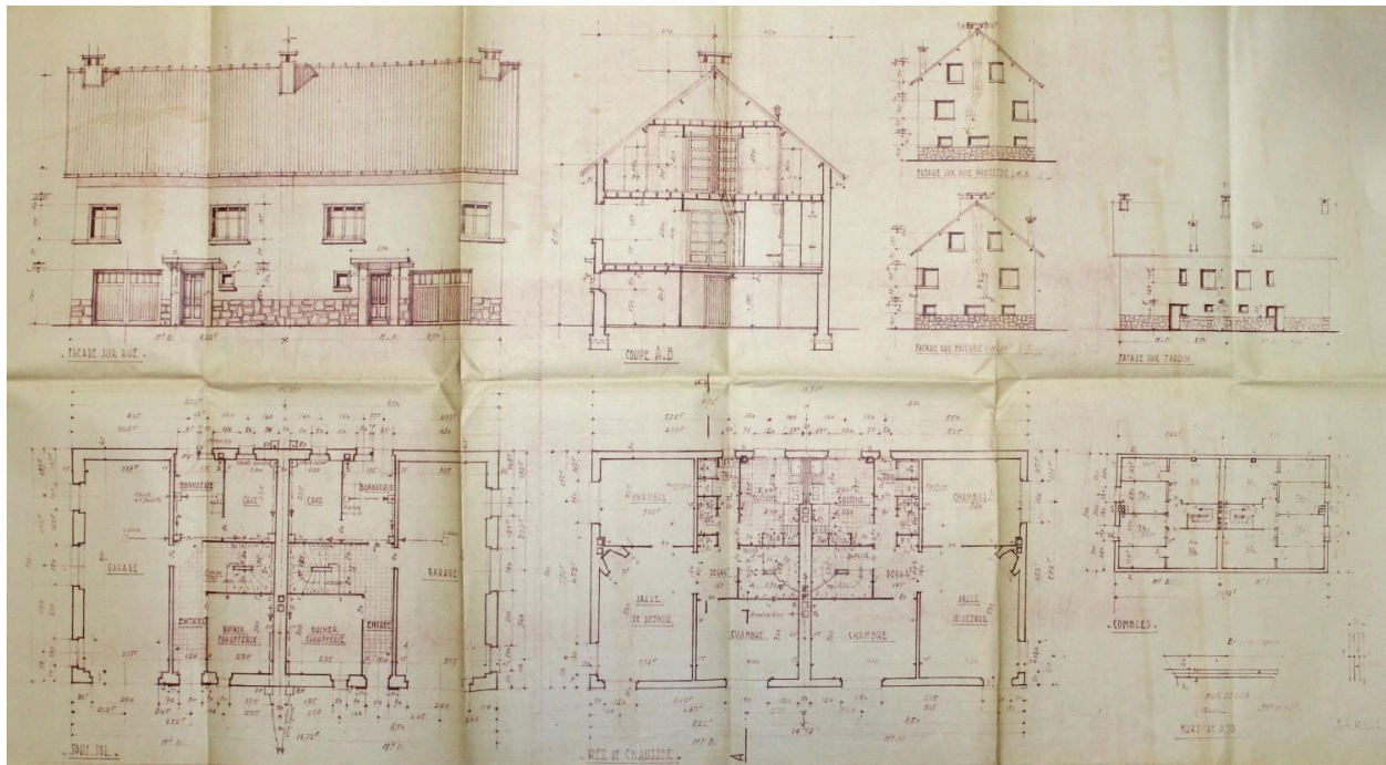
Aurillac, cité des Camisières, maisons jumelées n° 2 et 4 rue de la Santoire, plans, élévations et coupes, juin 1954, Pierre Terrisse architecte (Archives municipales d'Aurillac, 135 W 45, permis de construire n° 1434 et 1435).
