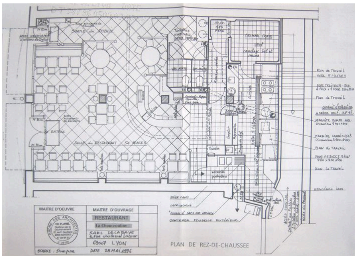
Plan du RDC, Restaurant La Choucroutine, 6 rue Challemel Lacour, 28 mai 1996 par Pluriel architecte échelle 1/20. (Arch. mun. Lyon)
