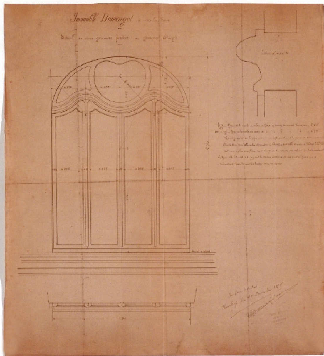
Détail d'une grande fenêtre
