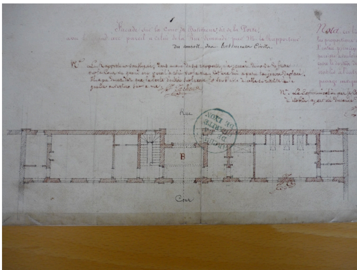
Plan du bâtiment de la porte d'entrée, 1826 (détail de la coupe). Plan AC Lyon. Fonds des HCL ; 2OP682
